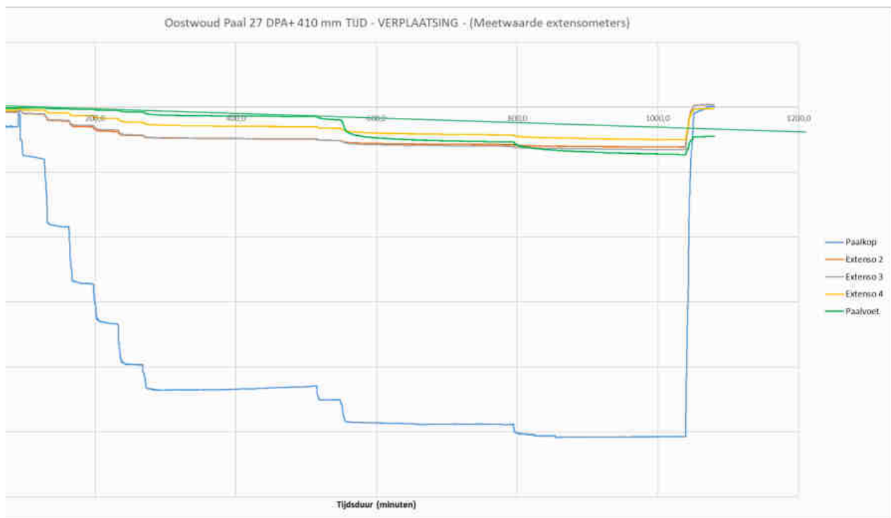
FIGUUR 25 CORRECTIE MEETRESULTATEN BIJ SLIPPEN SENSOR
